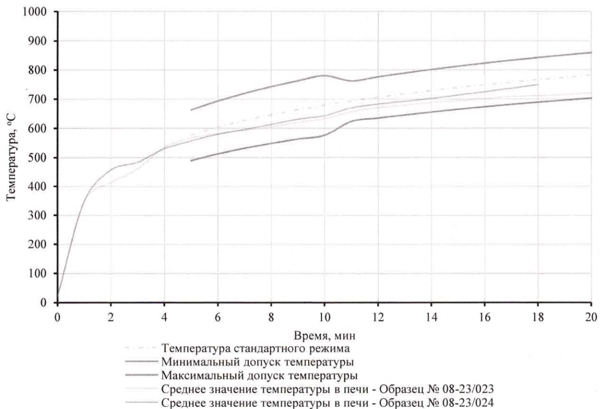
Рис. 5 Температура в печи при испытании образцов № 08-23/023 и № 08-23/024
