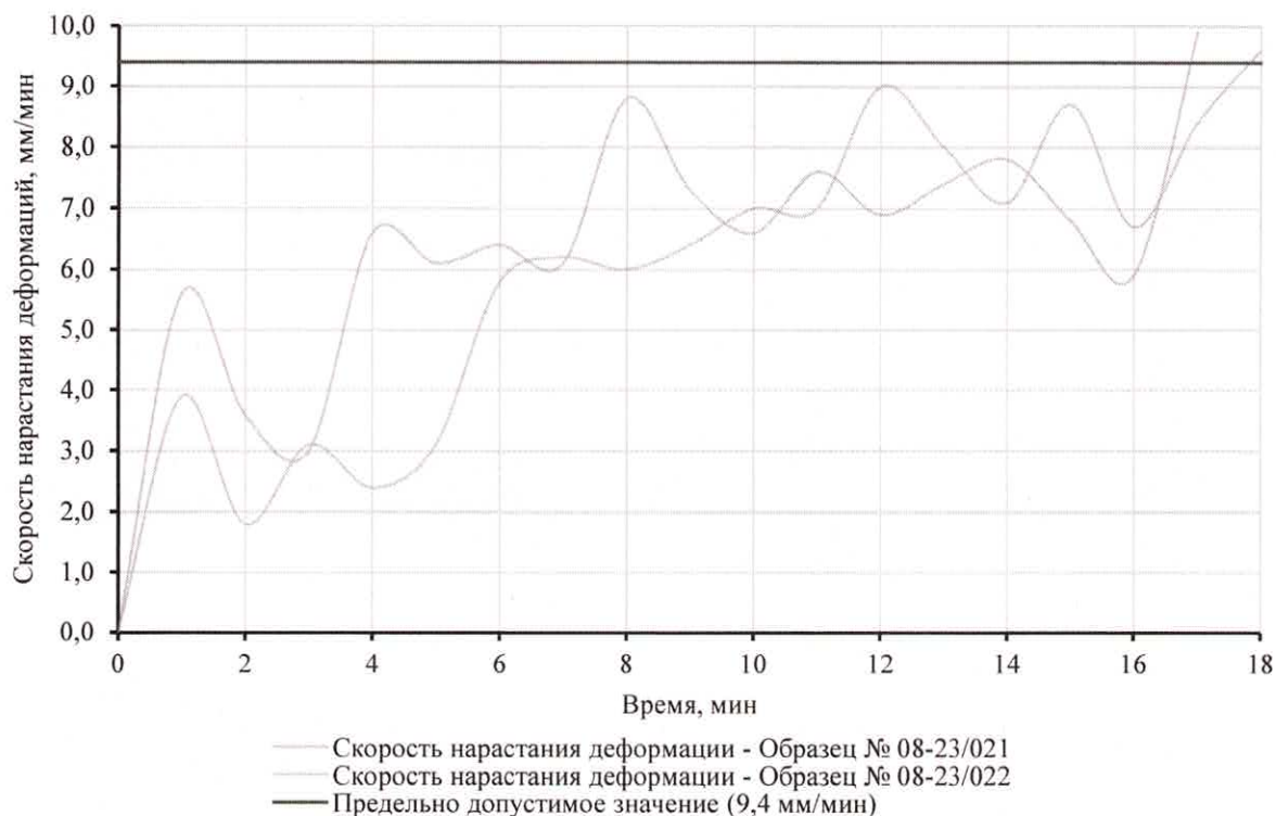
Рис. 4 График скорости нарастания деформации при испытании образцов № 08-23/021 и № 08-23/022
