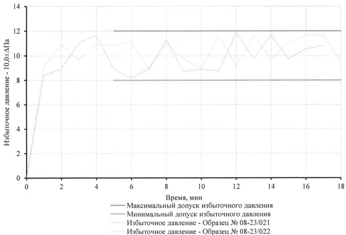
Рис. 2 График избыточного давления при испытаниях образцов № 08-23/021 и № 08-23/022
