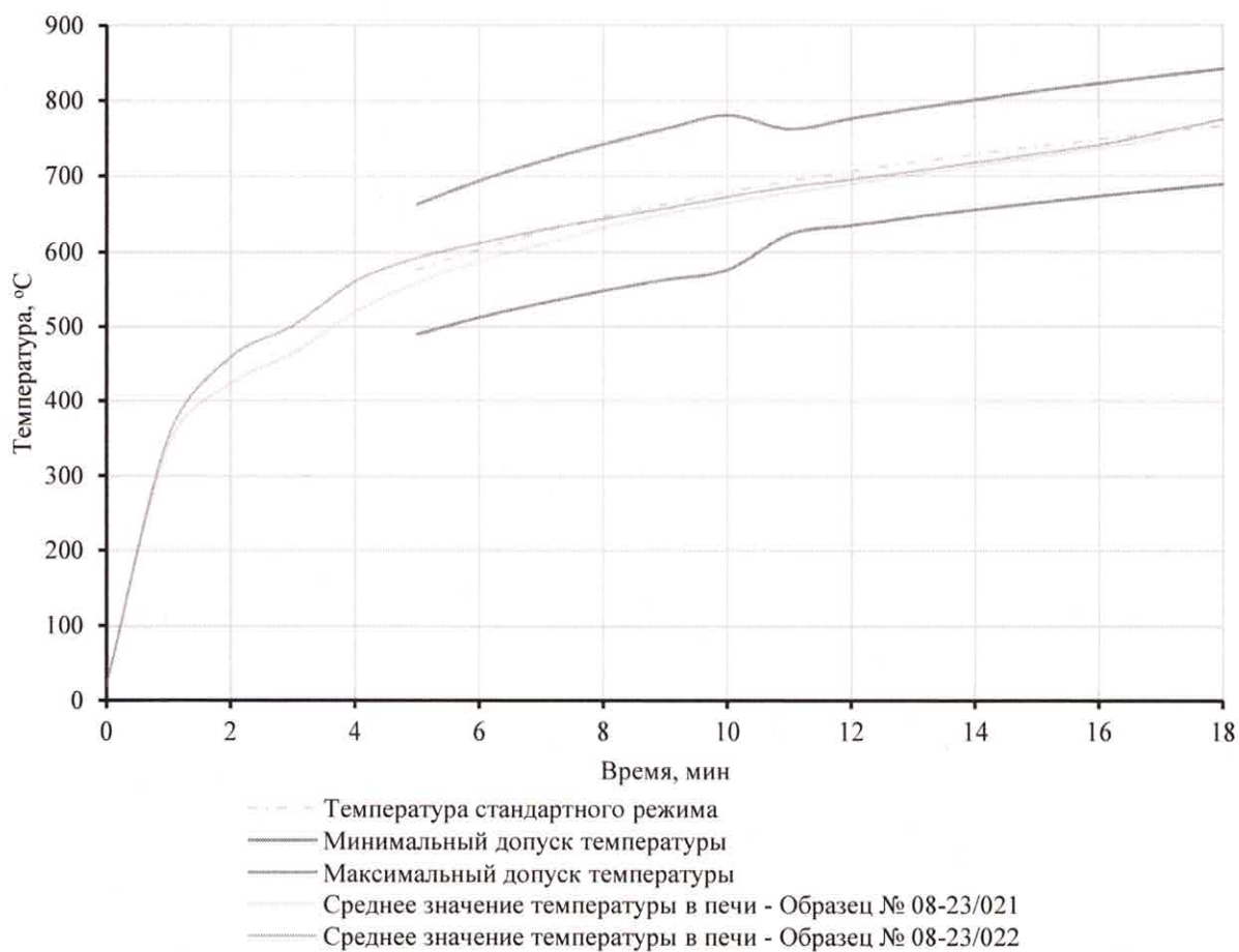
Рис. 1 Температура в печи при испытании образцов № 08-23/021 и № 08-23/022
