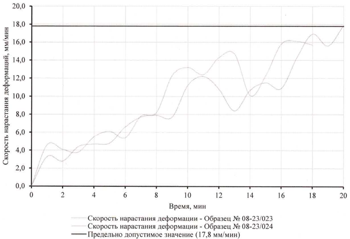
Рис. 8 График скорости нарастания деформации при испытании образцов № 08-23/023 и № 08-23/024
