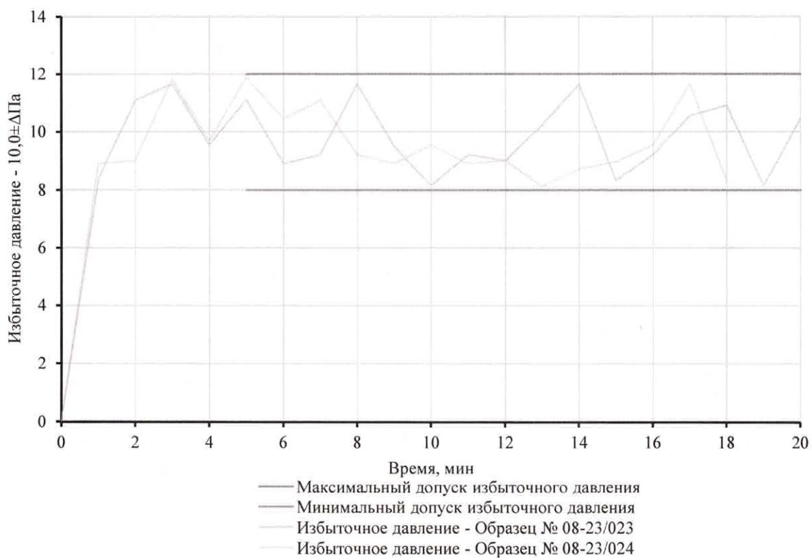
Рис. 6 График избыточного давления при испытаниях образцов № 08-23/023 и № 08-23/024
