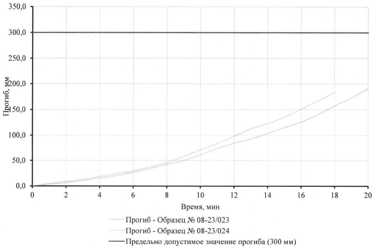
Рис. 7 График роста прогиба при испытании образцов № 08-23/023 и № 08-23/024
