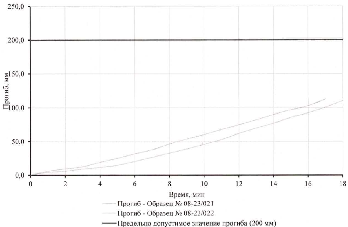
Рис. 3 График роста прогиба при испытании образцов № 08-23/021 и № 08-23/022
